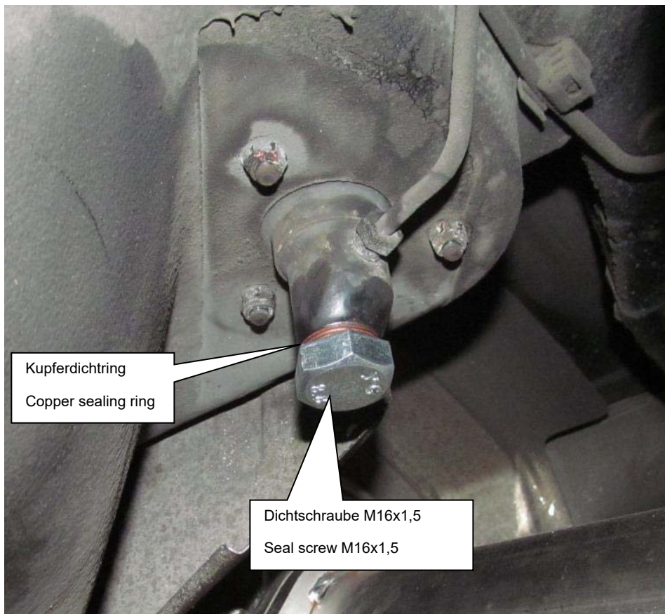
Dichtschraube M16x1,5 Seal screw M16x1,5
